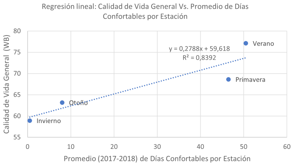
Gráfico 3: Regresión lineal simple para las variables Calidad de Vida General y el promedio de Días confortables en función de las estaciones del año, para el periodo 2017-2018.
